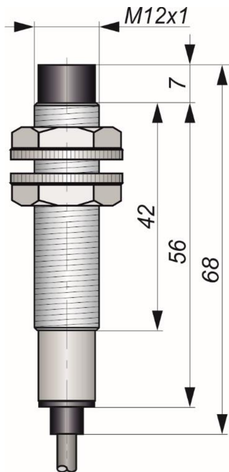
Габаритный чертеж
