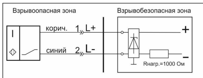
Схема соединения
